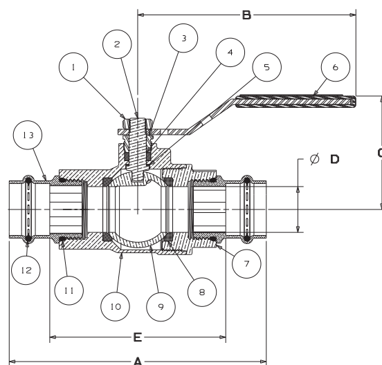
PC-585-66-LF P x P
