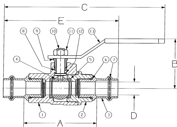
PC-585-70-66 P x P
