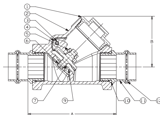
PC-413-Y-LF Press x Press
