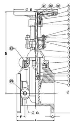
F-607-RW Flg x Flg
