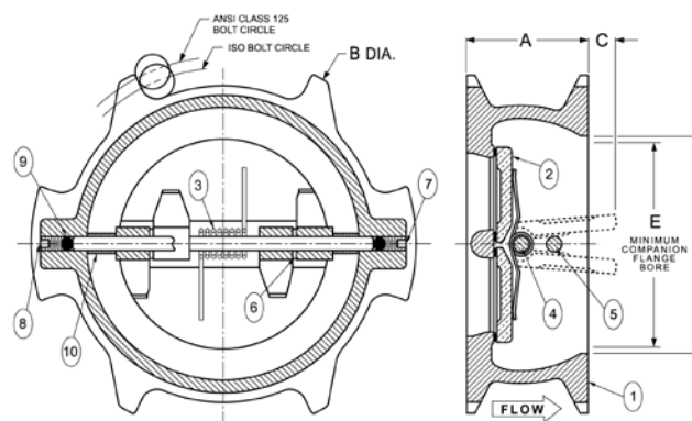
W-920-W Wafer
