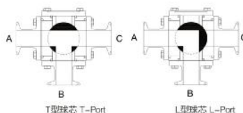
T型球芯 T-Port
