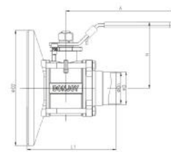
罐底三片式无旁通球阀 NO. VQW120S1-06
