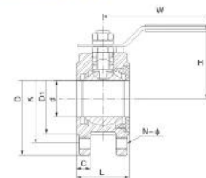
主要外形尺寸 Main size
