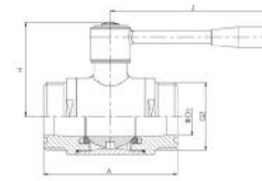
SMS螺纹 NO.SMS-VOC130S1
