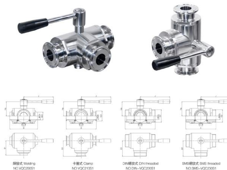
手动球阀尺寸图 Manual ball valve Dimension
