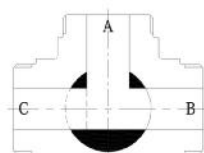
T型球芯 T Port
